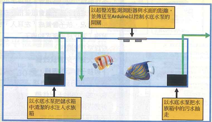
● 換水系統的原理及運作展示圖。
